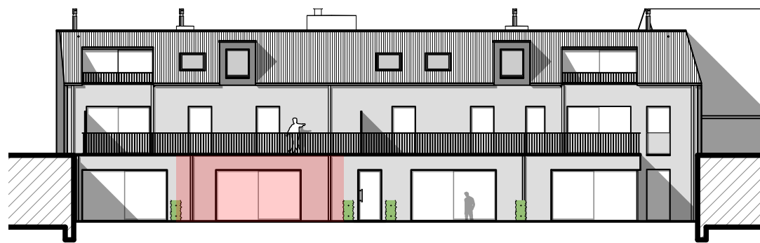
ACHTERGEVEL
